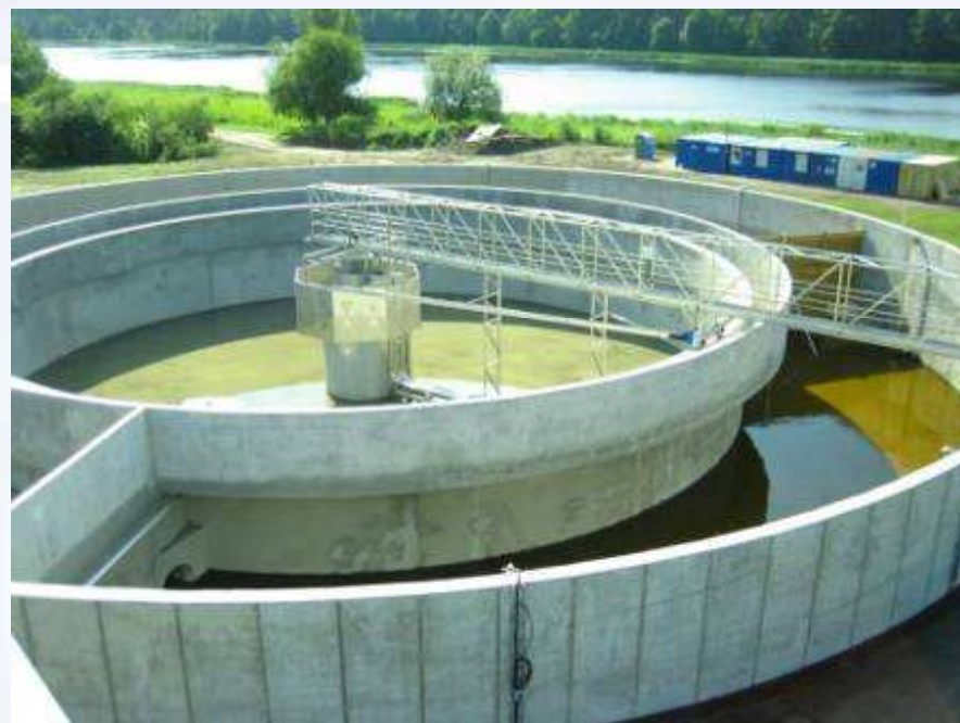
Pildil: reoveepuhastite ehitus Jurmala Lätis, ehitaja Abagars SIA
